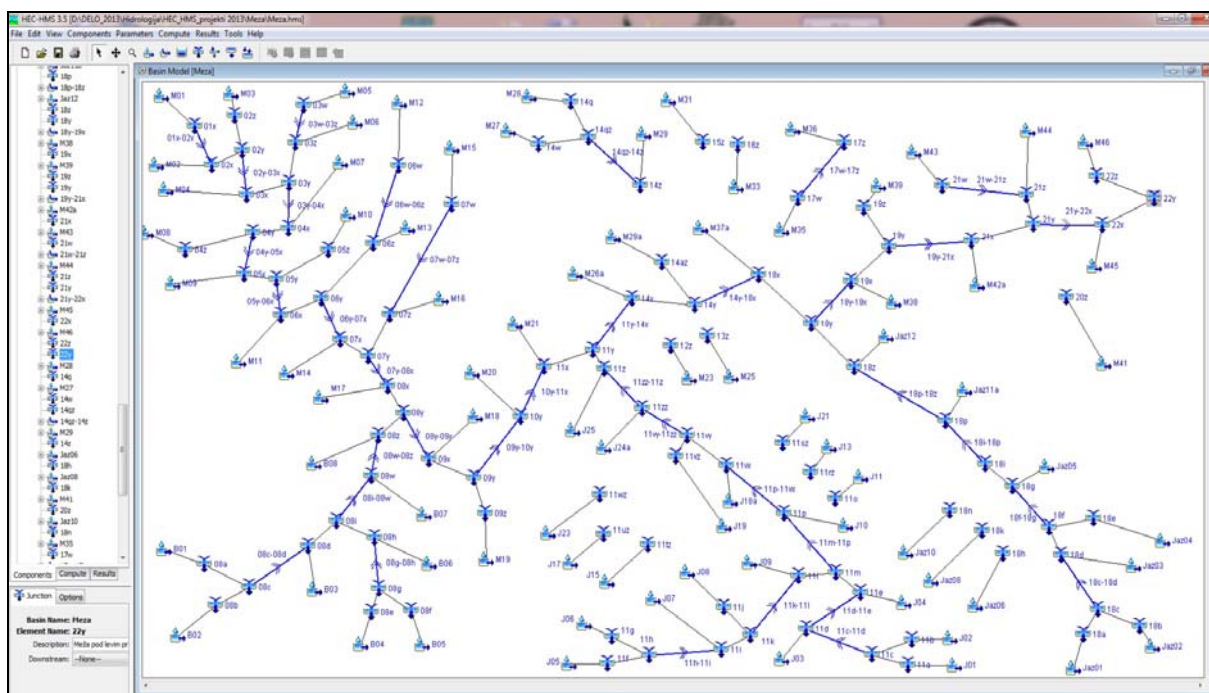
Slika 2: Hidrološki model porečja Meže s pritoki
